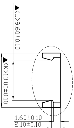
A部詳圖: (塑柱: 2/1)
