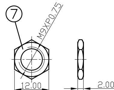
NUT
