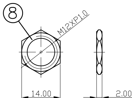
NUT
