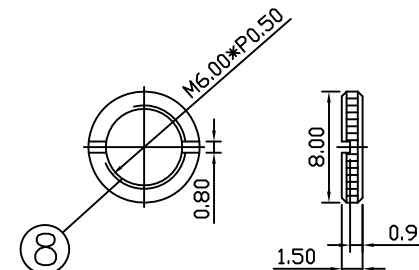
NUT
