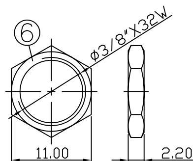
Nut
