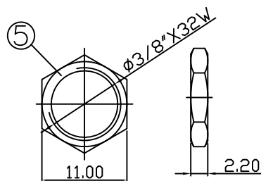
NUT
