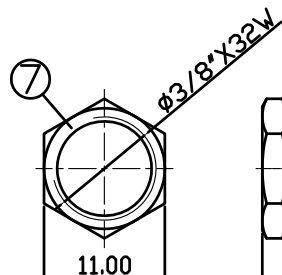
NUT
