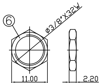
NUT
