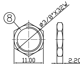
NUT
