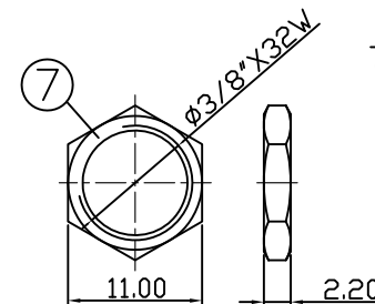
NUT
