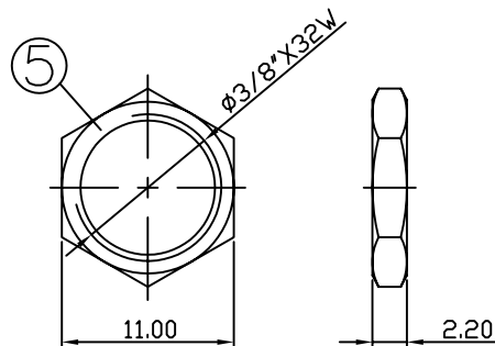
NUT
