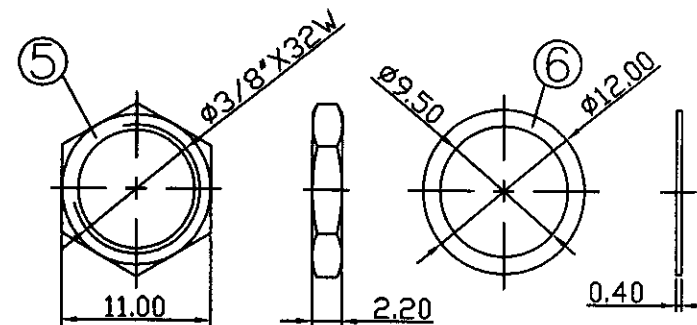
Nut Washer
