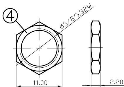
Nut
