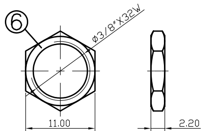
NUT
