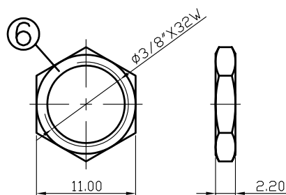
NUT
