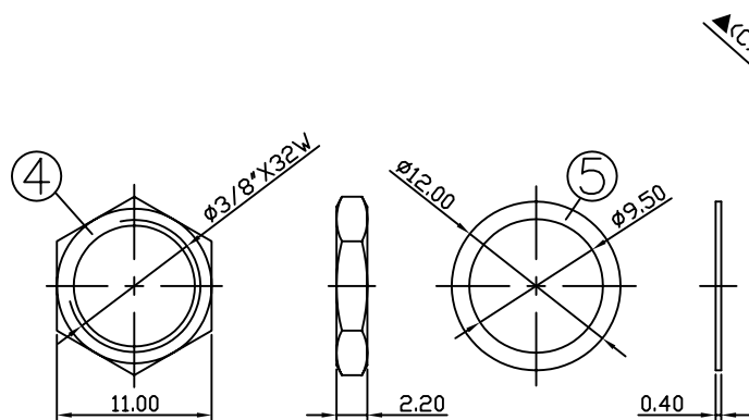
NUT
