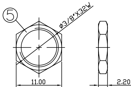
NUT
