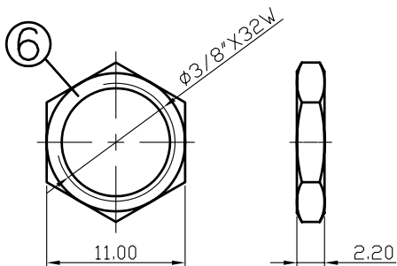
NUT
