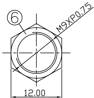
Nut
