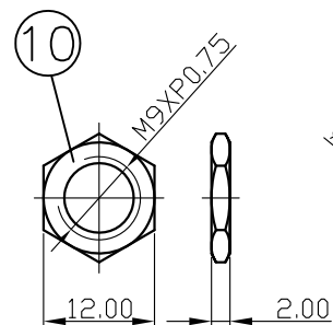
NUT
