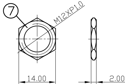
NUT
