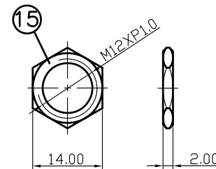
NUT
