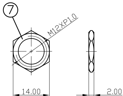
NUT
