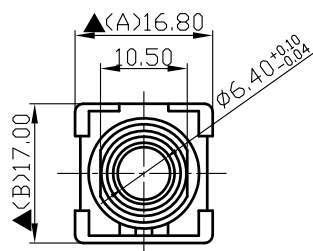
NUT
