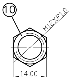
NUT
