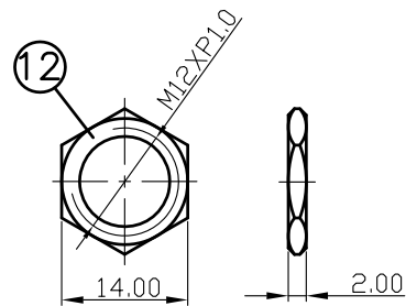
NUT
