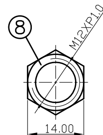
NUT
