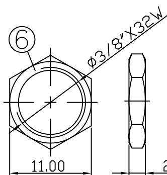
Nut
