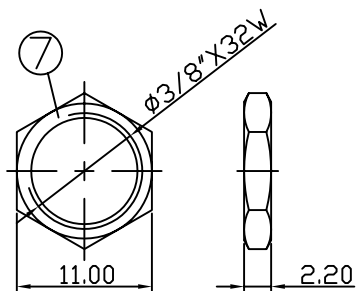
Nut
