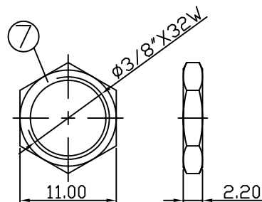
Nut
