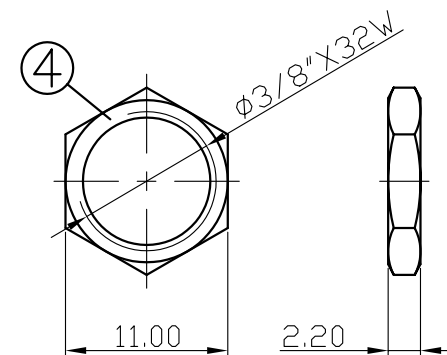
NUT
