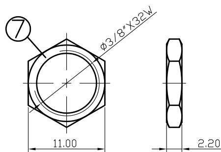
NUT
