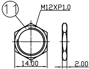
NUT
