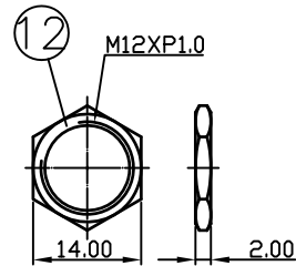
NUT
