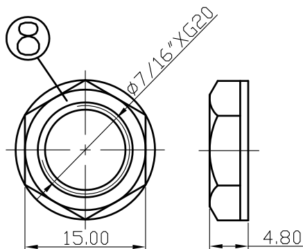
NUT
