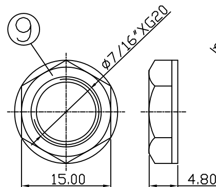
NUT
