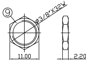
NUT
