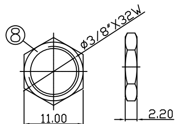
NUT
