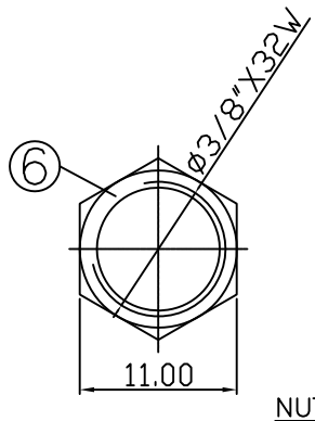
NUT
