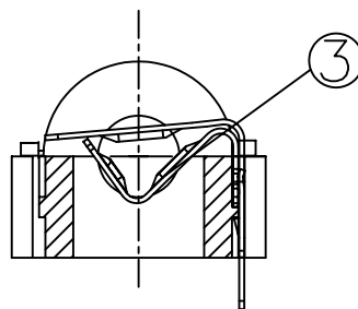
A-A剖面
