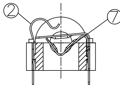
A-A剖面
